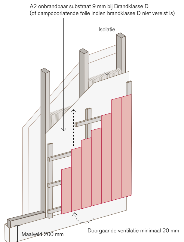
Dubbele belatting bij verticale toepassing van gevelbekleding
